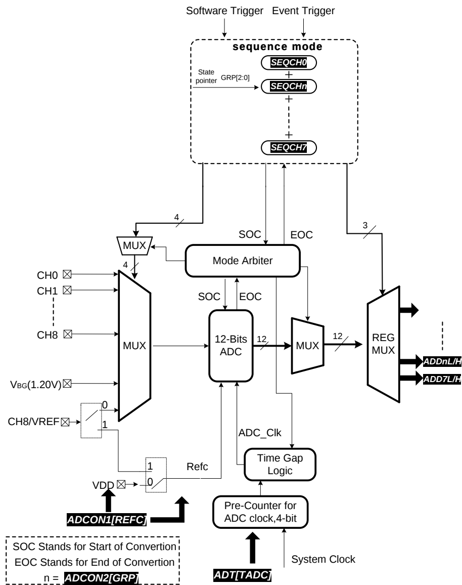
图9.9-1 ADC模块图
