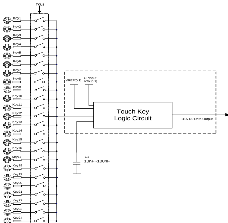
系统框图
