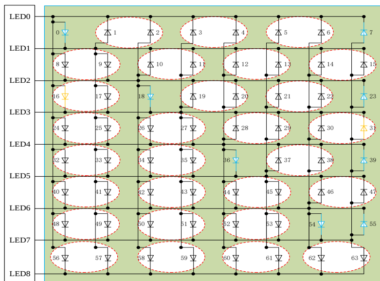
LED 8*8 点阵图
