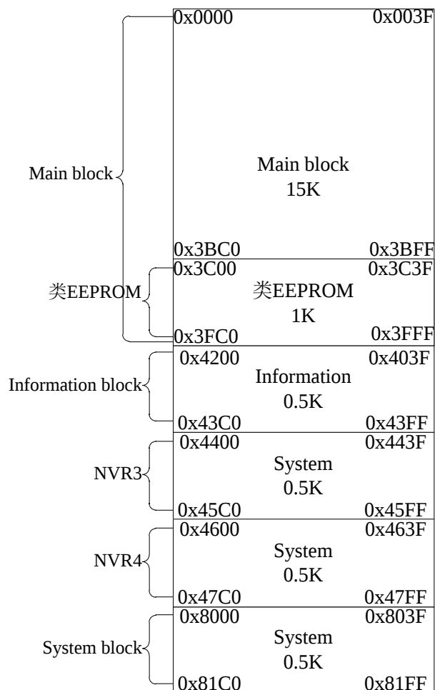
Flash 程序存储器地址分配结构图
