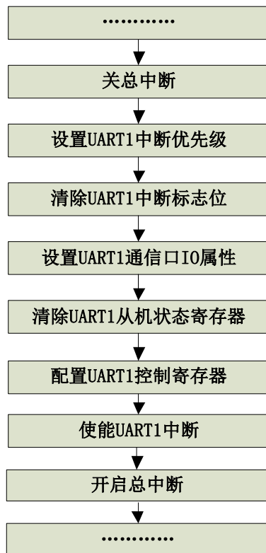
UART1 初始化配置流程图
