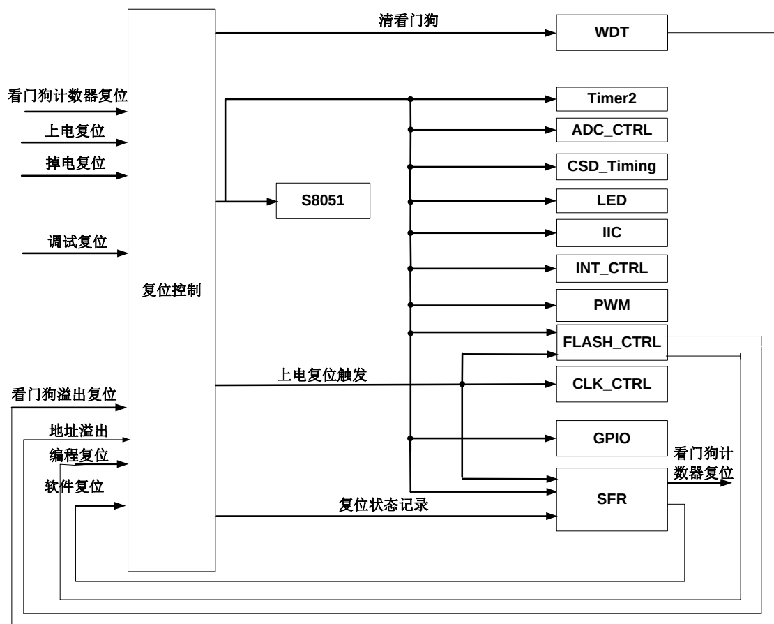
复位方框图
