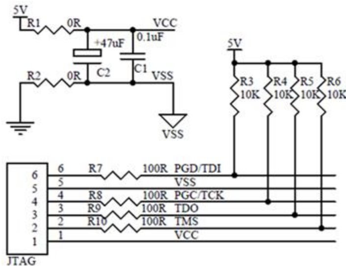
JTAG 电路连接参考图
