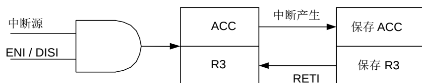
图 6-13 中断保存框图
