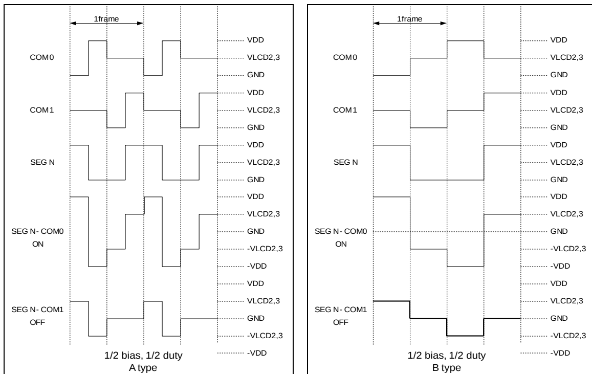
图. 6-16 1/2 偏压, 1/2 占空比的LCD波形
