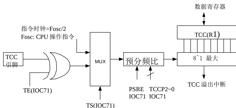
图. 6-4(a) TCC 结构框图
