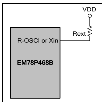
图 6-9 内部电容振荡器模式电路
